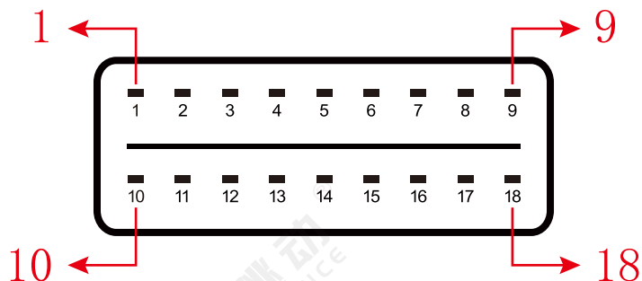
KDS3.1尿素泵侧接头针脚图
